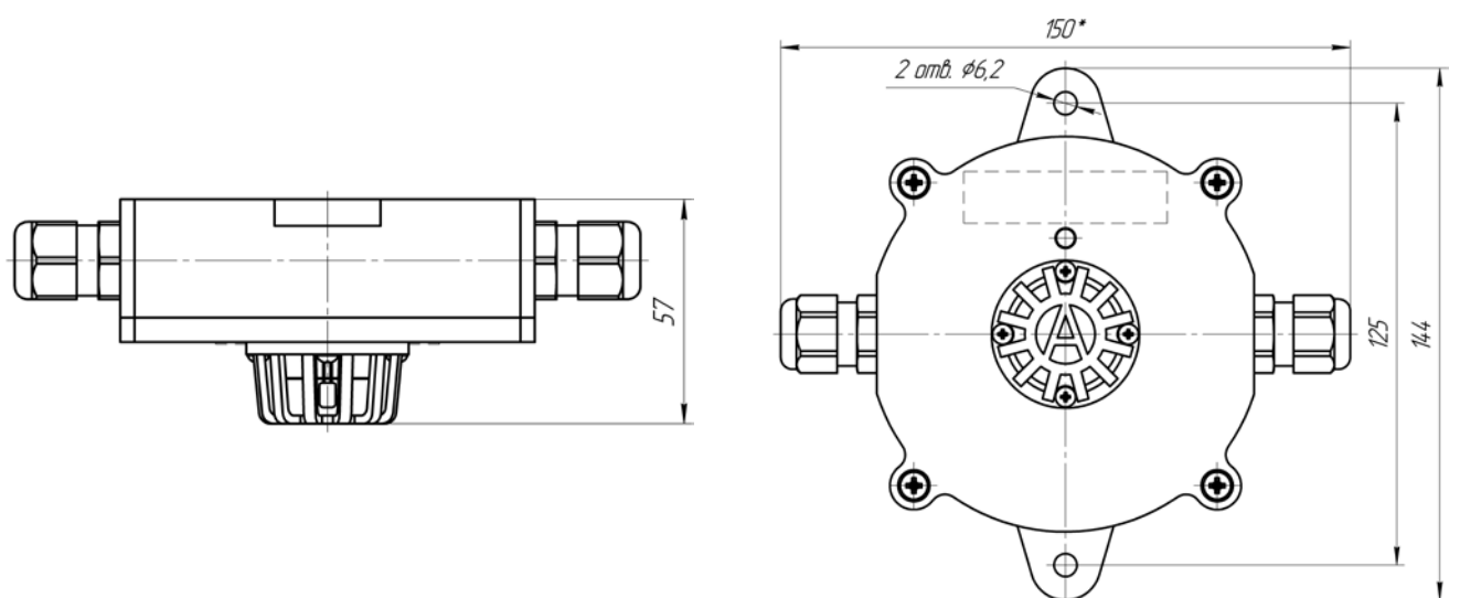
Рис.3 – Внешний вид, габаритные и установочные размеры извещателей СПТТА, СПТТА-В в корпусе К2, размеры в мм.
