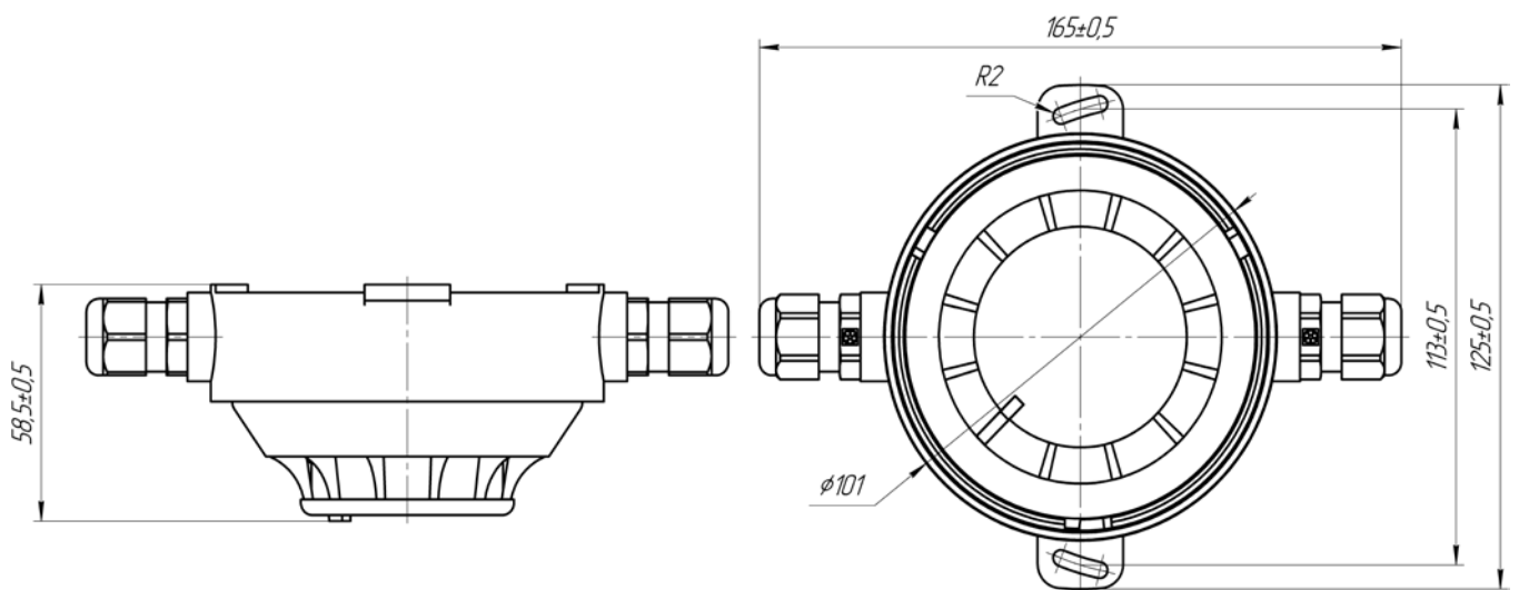
Рис.3 – Внешний вид, габаритные и установочные размеры извещателей СПТТА, СПТТА-В в корпусе К2, размеры в мм.
