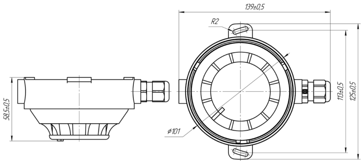
Рис.2 – Внешний вид, габаритные и установочные размеры извещателей СПТТА, СПТТА-В в корпусе К1, размеры в мм.
