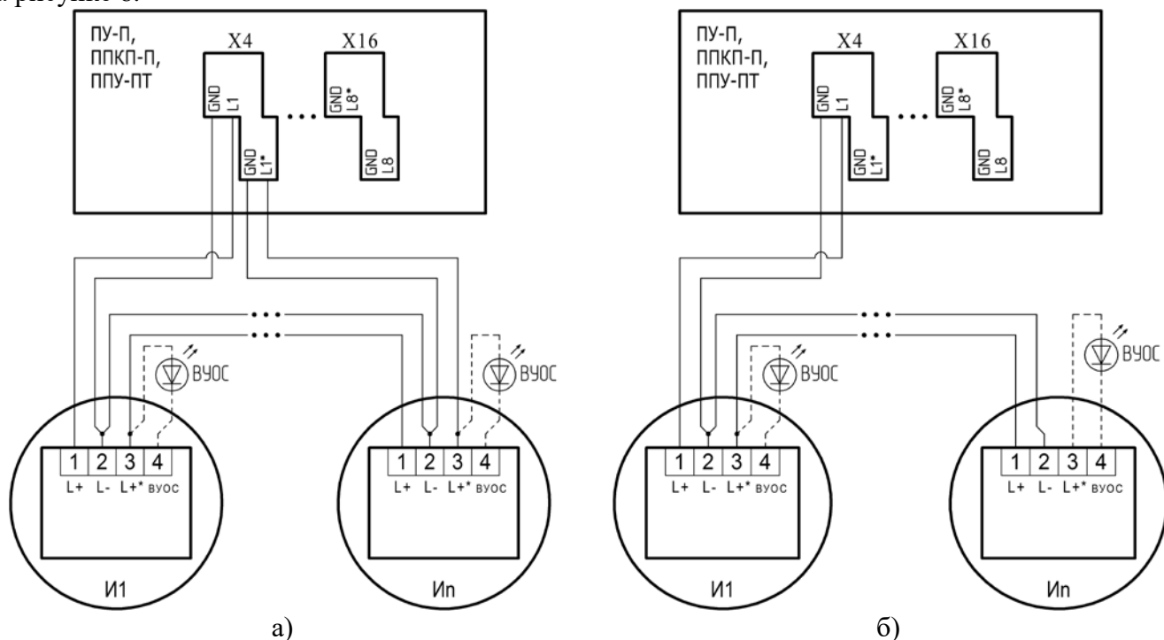
Рис.6 – Типовая схема подключения извещателей СПТТА и СПТТА-01 к ППКП АСПС, (а) кольцевое включение, (б) лучевое подключение.
