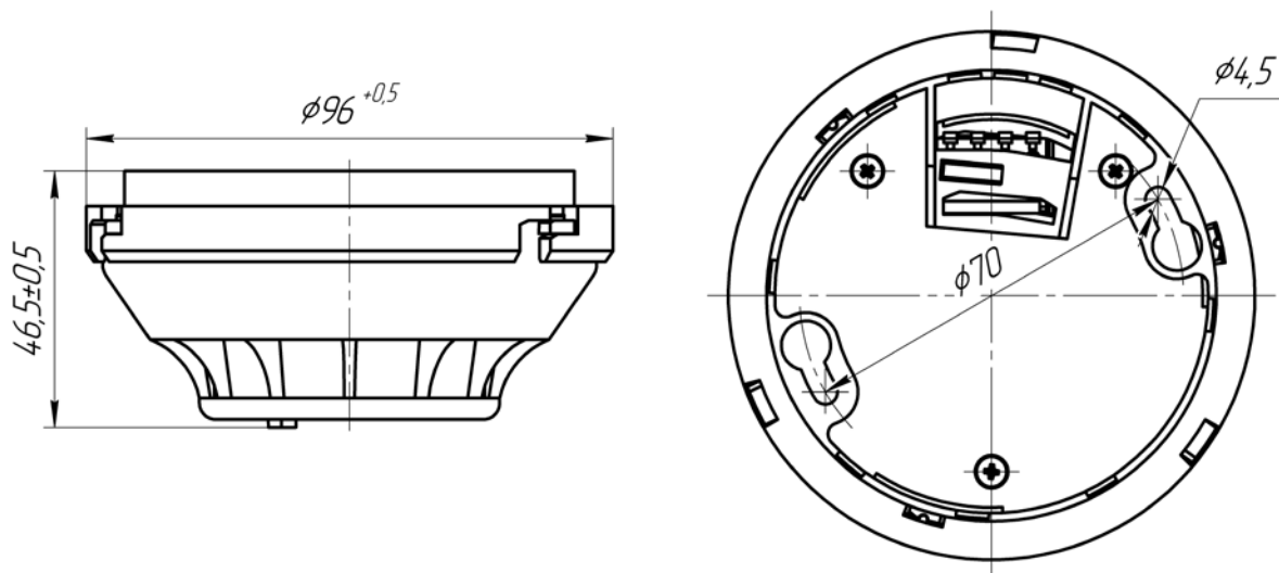
Рис.1 – Внешний вид, габаритные и установочные размеры извещателей СПТТА и СПТТА-В с установленной розеткой Р-96, размеры в мм.
