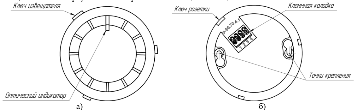
Рис.5 – Конструкция извещателя, (а) - извещатель, (б) - розетка.
