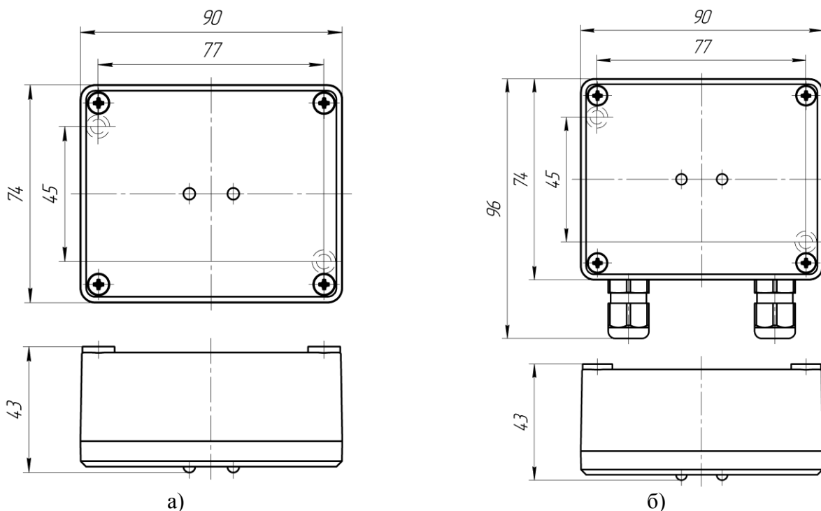
Рис.1 Внешний вид, габаритно-установочные размеры ИКЛ (а), ИКЛ-01 (б), размеры в мм.
